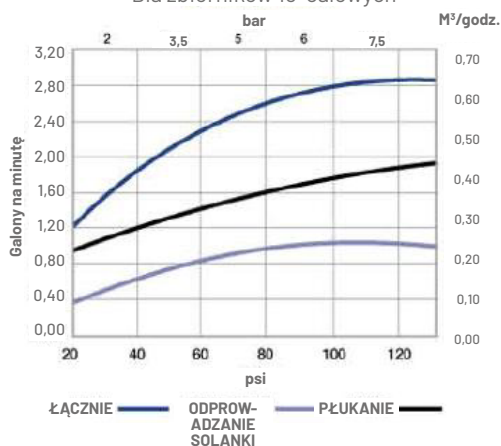
Injektor „Q” (fioletowy) Dla zbiorników 18-calowych
