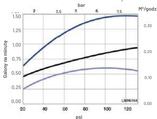
Injektor „L” (pomarańczowy) Dla zbiorników 13- i 14-calowych
