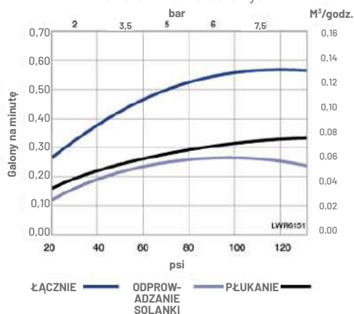
Injektor „K” (różowy) Dla zbiorników 12-calowych
