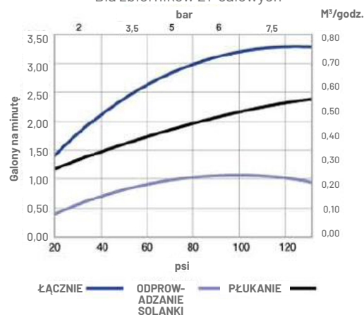
Injektor „R” (ciemnoszary) Dla zbiorników 21-calowych
