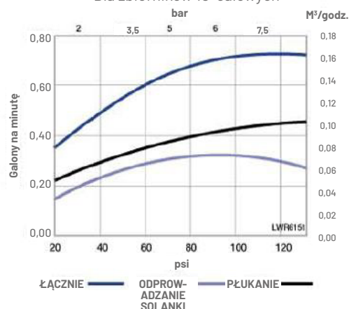
Injektor „L” (pomarańczowy) Dla zbiorników 13- i 14-calowych
