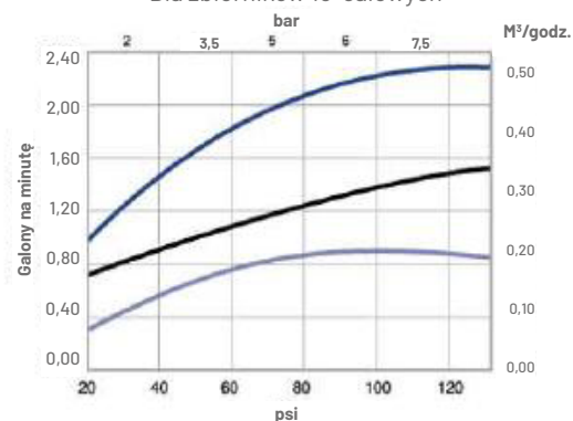
Injektor „N” (zielony) Dla zbiorników 16-calowych
