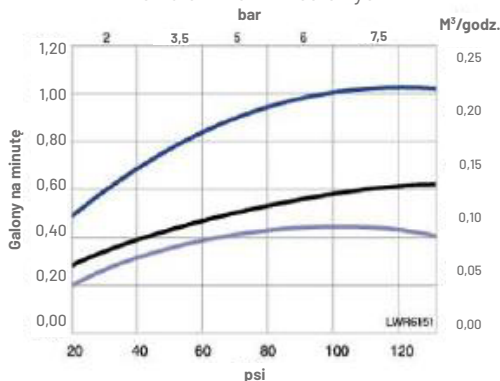
Injektor „K” (różowy) Dla zbiorników 12-calowych
