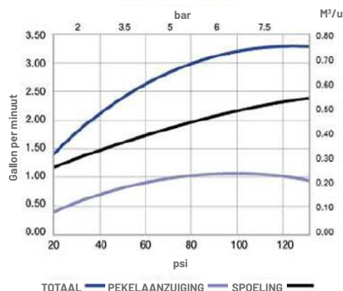
Injector "R" (donkergrijs) Voor tanks van 21 duims
