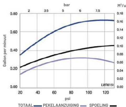
Injector "J" (lichtblauw) Voor tanks van 10 duims
