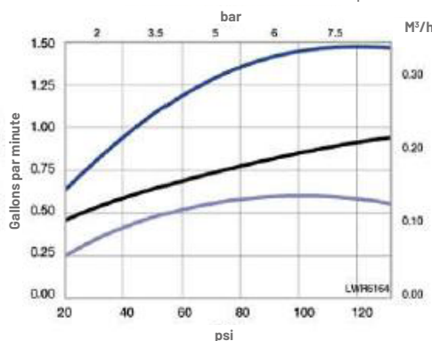
Injecteur "L" (orange) Pour les réservoirs de 13 et 14 pouces
