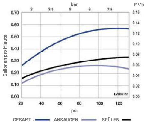
Injektor "H" (hell lila) für 9 Zoll-Tanks
