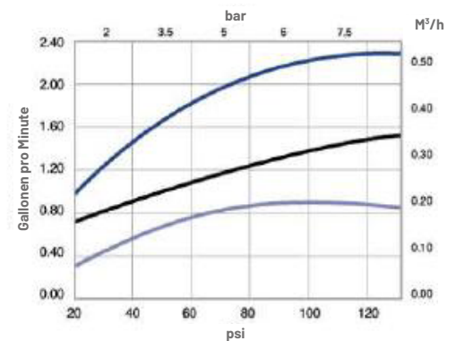
Injektor "R" (dunkel grau) für 21 Zoll-Tanks
