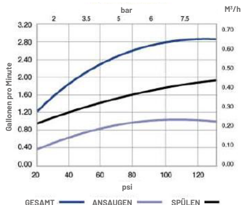
Injektor "Q" (lila) für 18 Zoll-Tanks
