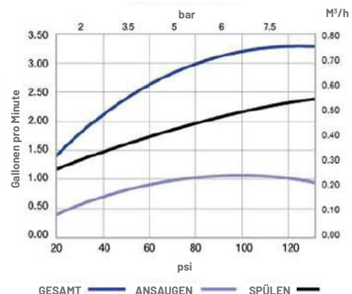
Injektor "R" (dunkel grau) für 21 Zoll-Tanks
