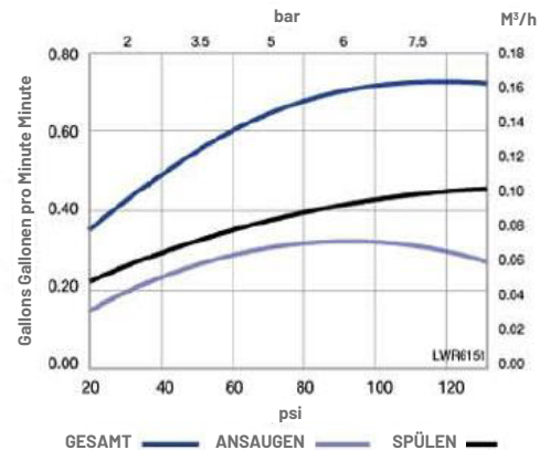
Injektor "J" (hellblau) für 10 Zoll-Tanks
