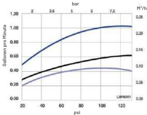
Injektor "Q" (lila) für 18 Zoll-Tanks
