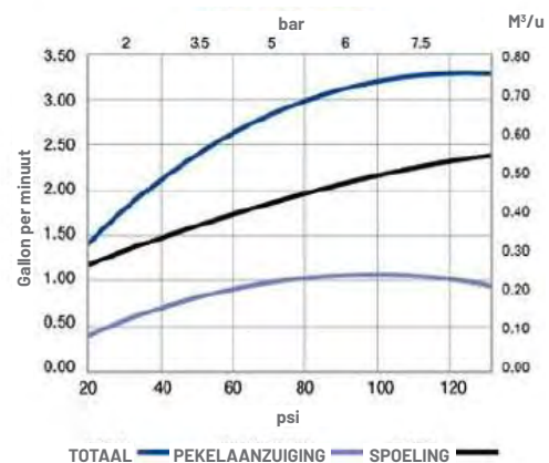
Injector "R" (donkergrijs) Voor tanks van 21 duims
